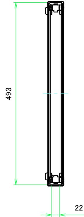
A-A (1:6)
